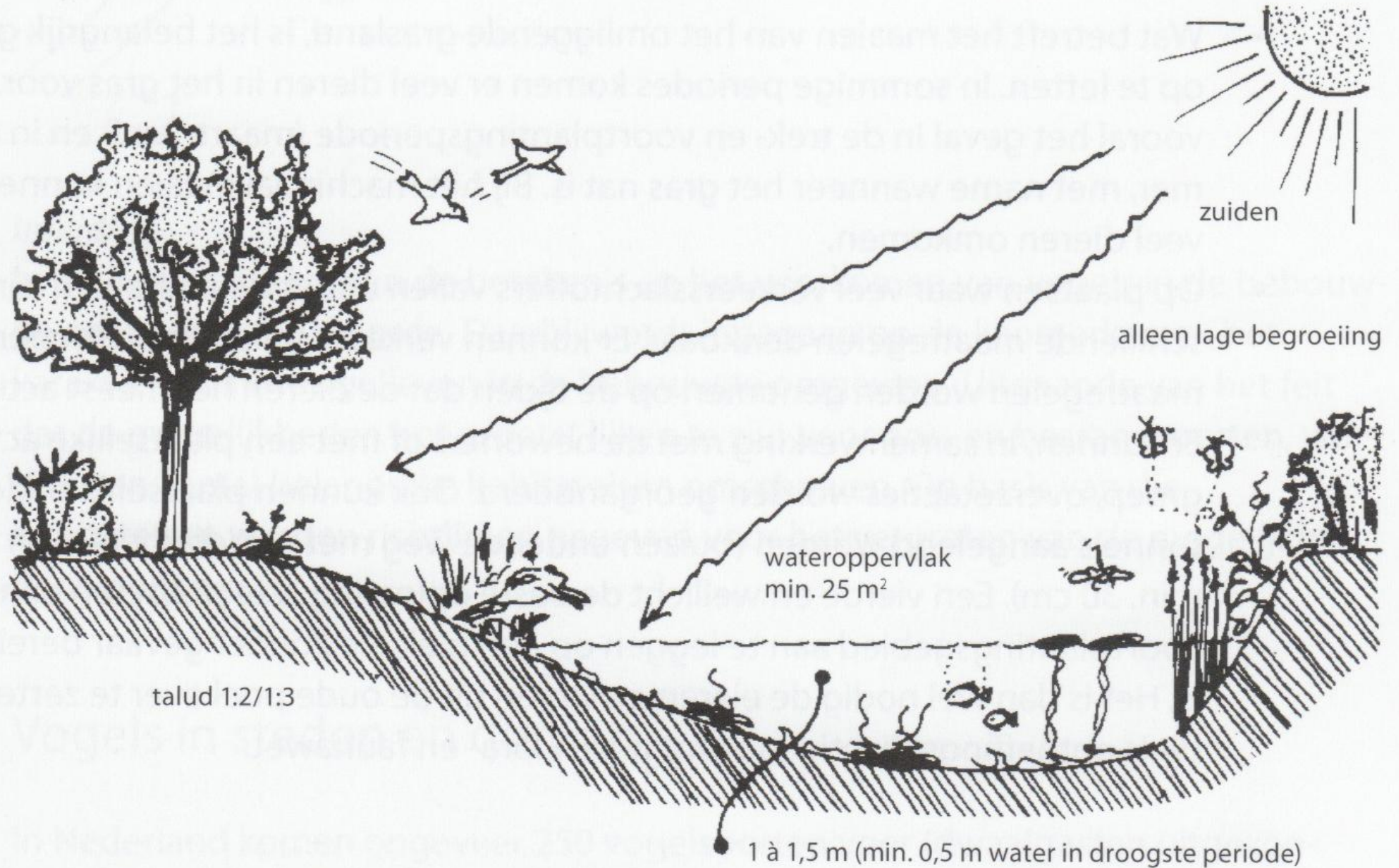
Schematische weergave van een goede poel (naar: Van Berkel & Steinhauer, 1988).
